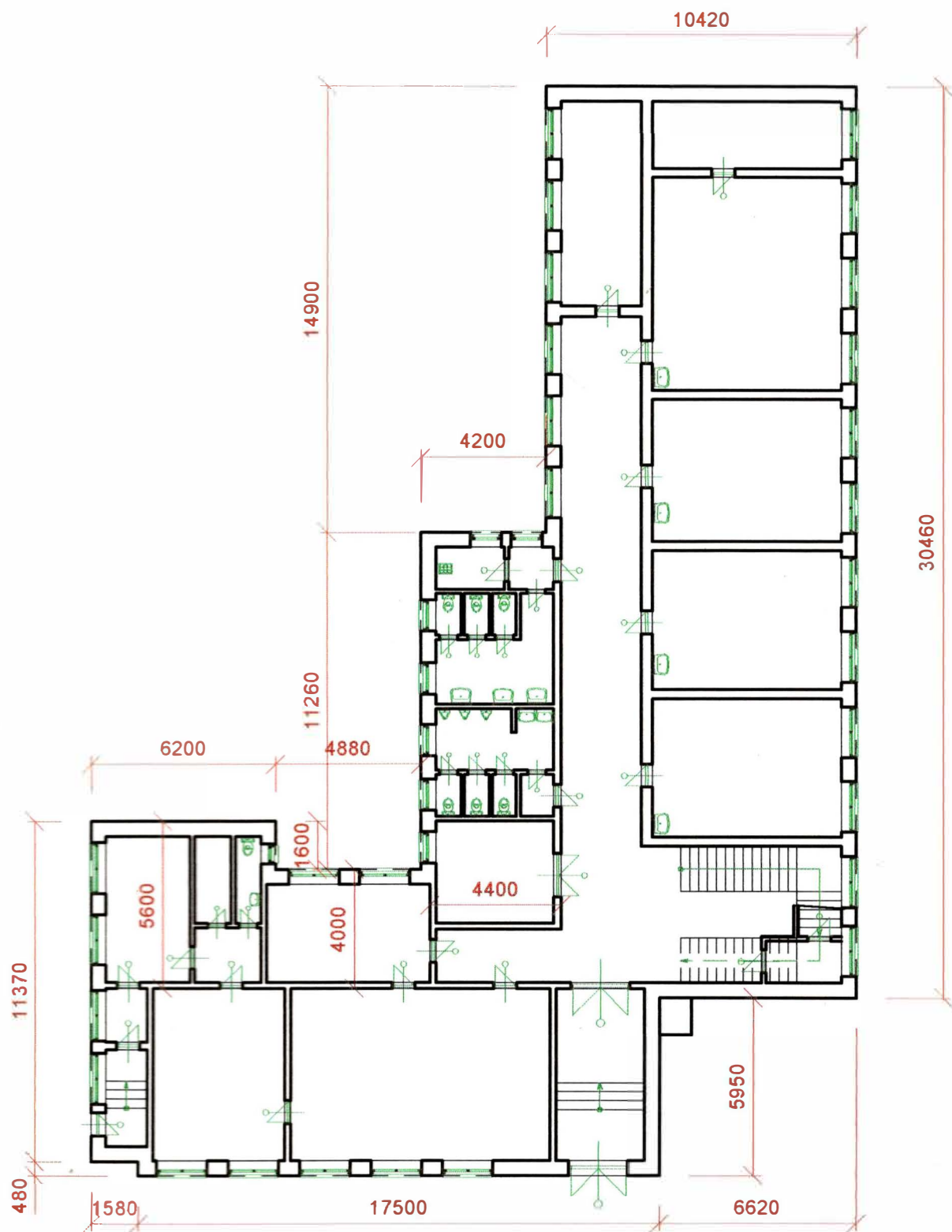
Príloha č.2 Budova školy súp.č.3280 na parc.č.5486/1 v k.ú.Petržalka Pôdorys 1.NP M 1 : 200
